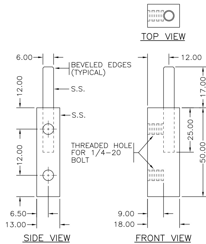
ITEM 12E (TOP DOOR HINGE - CABINET MOUNT)
