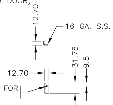
ITEM 11A (LOWER DOOR HINGE INSERT)
