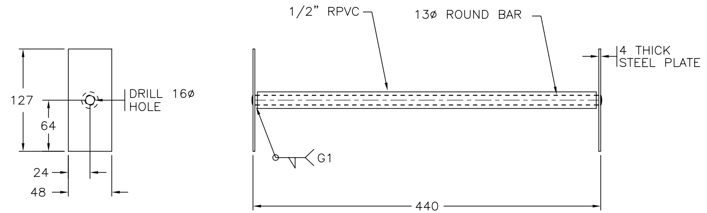
MID BRACE 1:5
