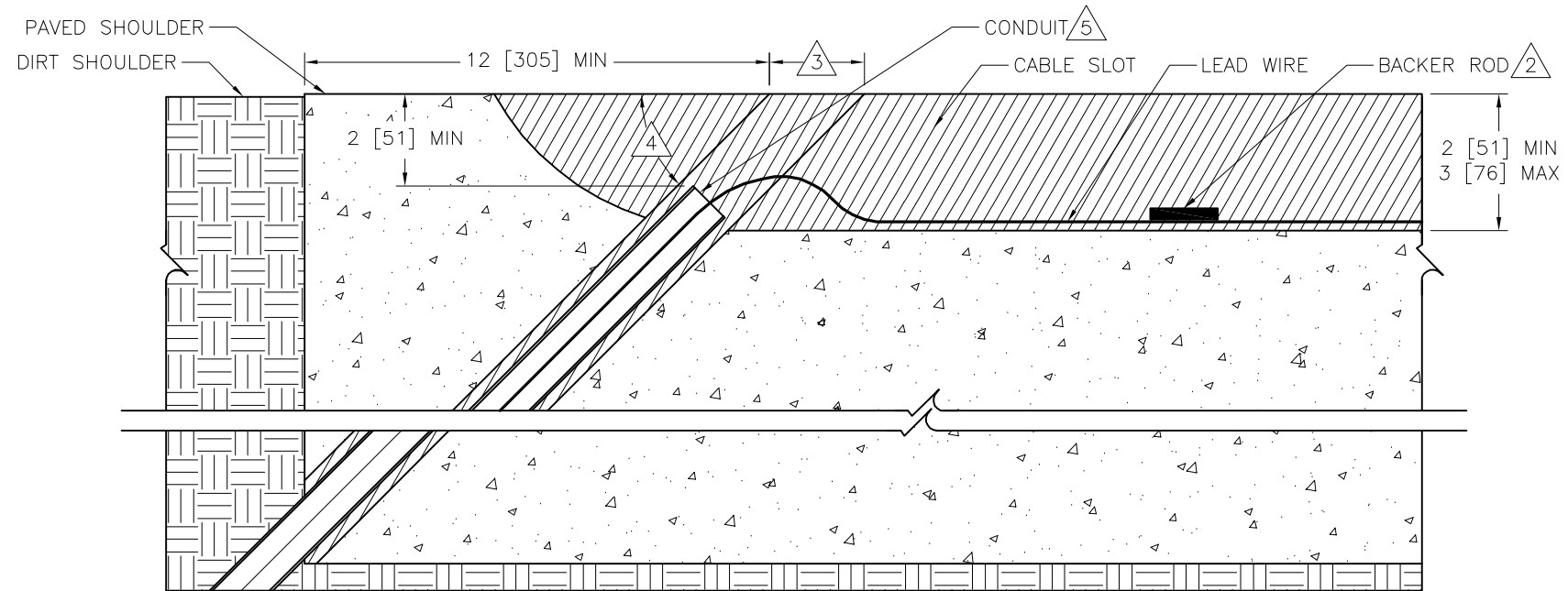
SECTION D-D
